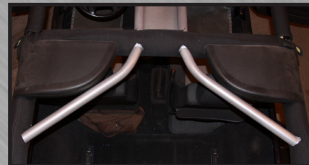
TJ & LJ ANGLE BARS 1997-2006 1997-2002 PART # RH1001-A 2003-2006 PART # RH1001-F $159.95
